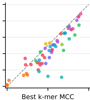
Evo2 (1B)
