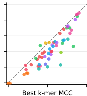
DNABERT-2
