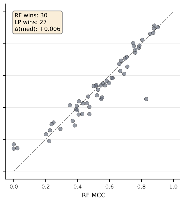
k-mer (k=6)
