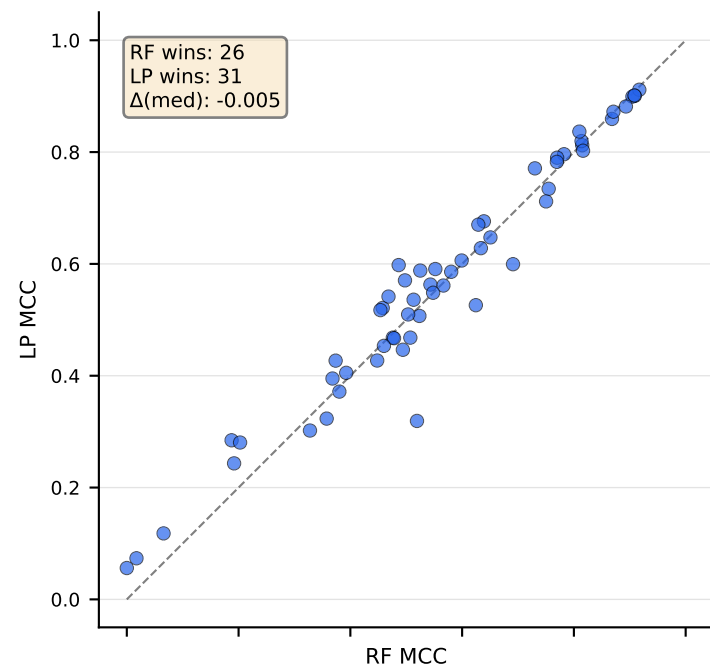
DNABERT-2
