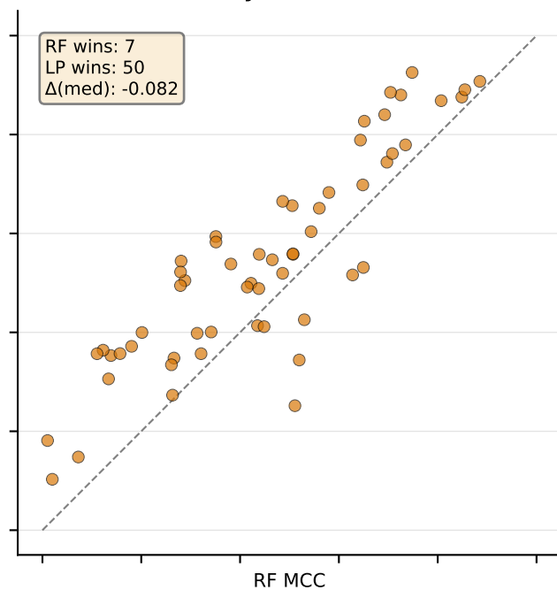
k-mer (k=6)
