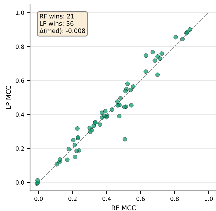
DNABERT-2
