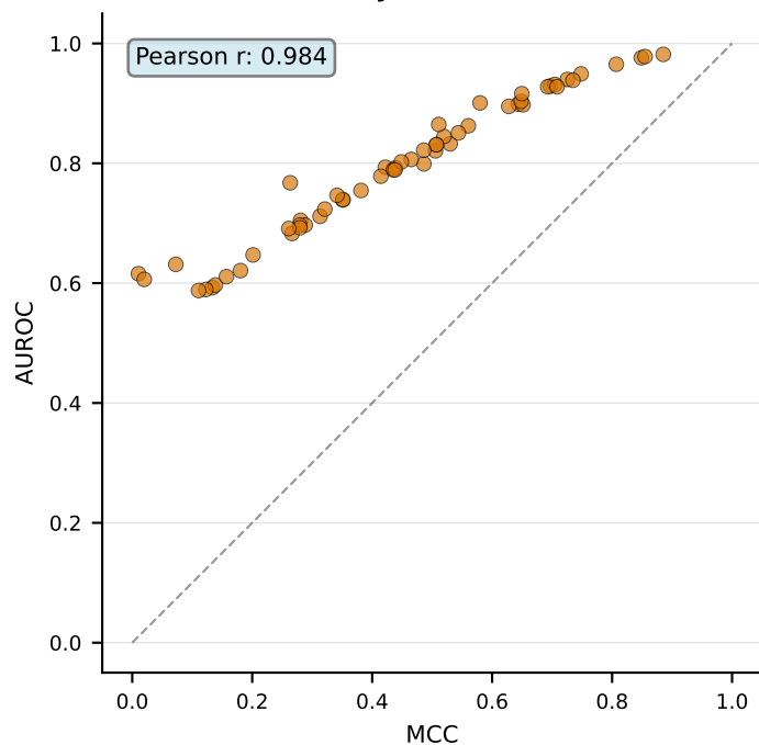
Caduceus
