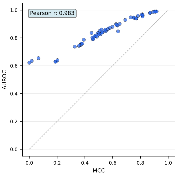
DNABERT-2
