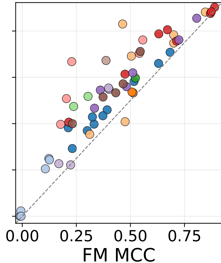
DNABERT-2
