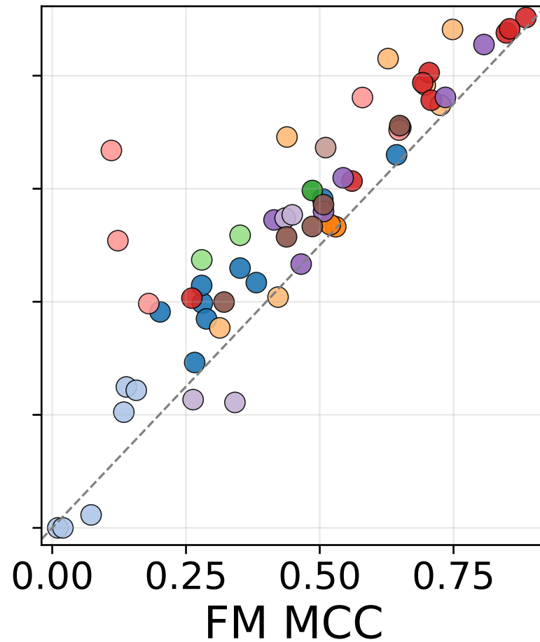
HyenaDNA-160k
