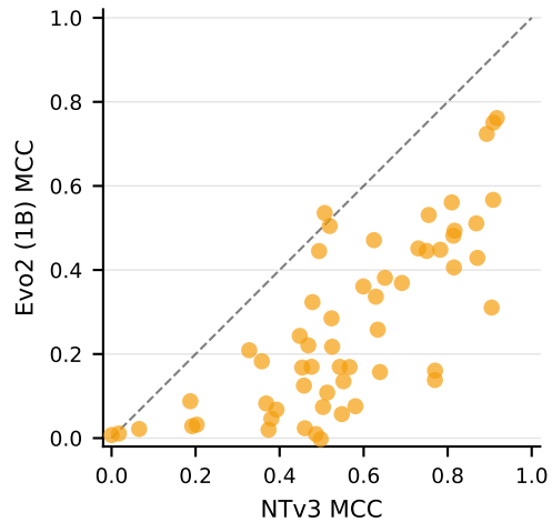
Evo2 vs NTV3 Evo2 wins: 2 | NTV3 wins: 55
