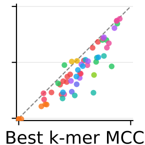
DNABERT-2
