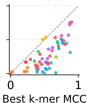
Evo2 (1B)
