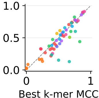
Caduceus
