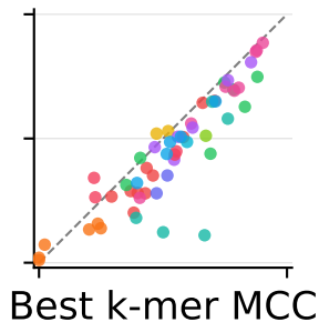
HyenaDNA
