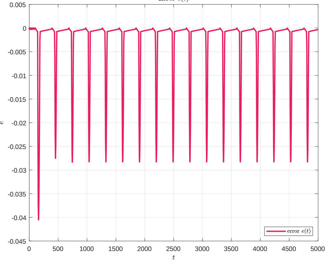
Error e(t)
