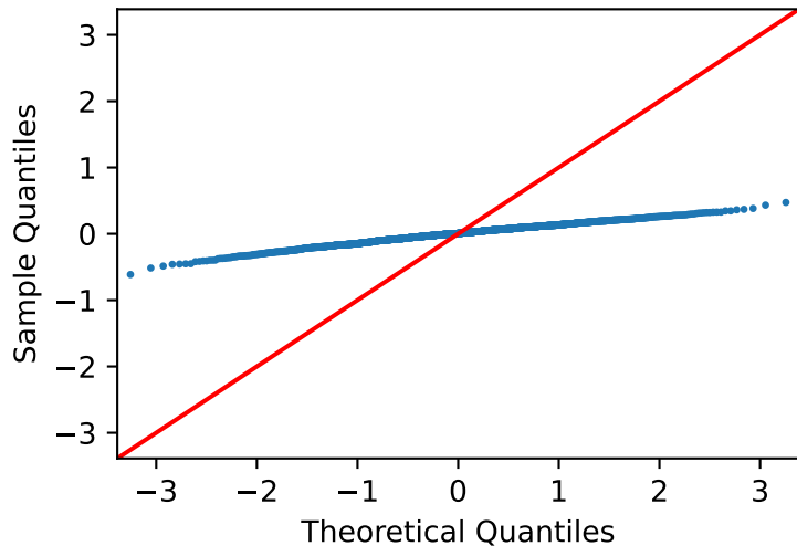
Normal Q--Q
