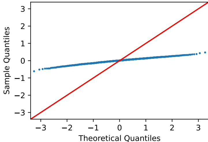
Normal Q--Q
