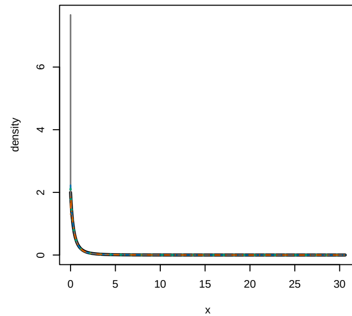
lomax_2, n=1000
