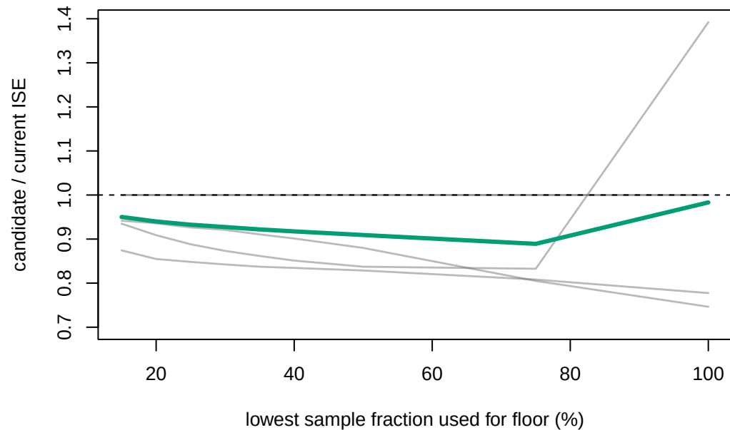
global ISE, n=1000
