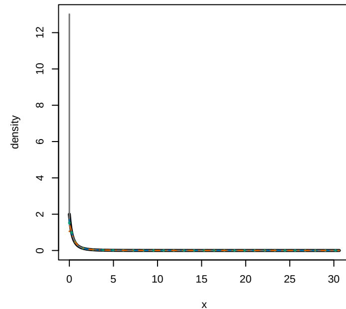
lomax_2, n=1000
