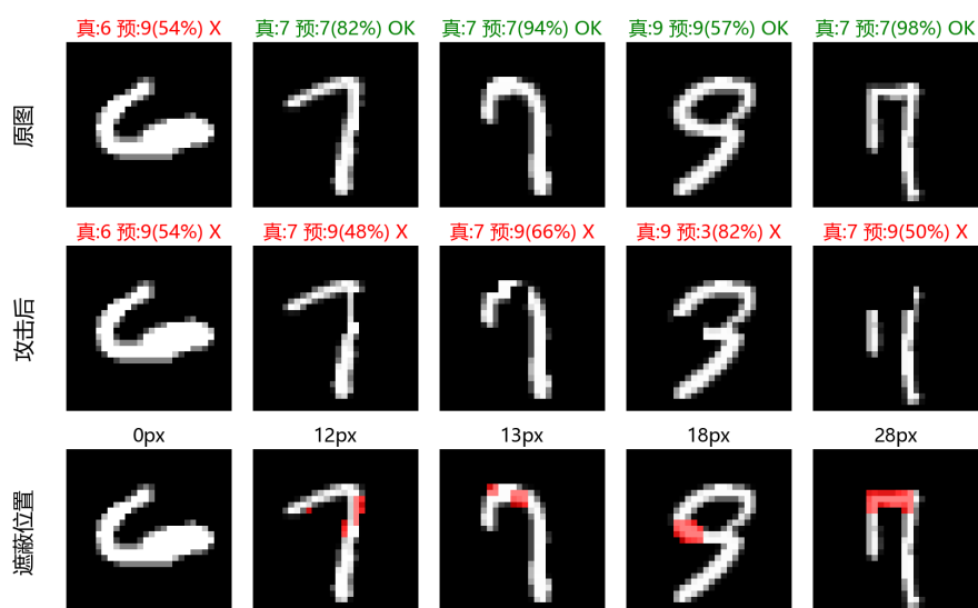
图 4.9 Adaptive-Saliency-AT 模型上的 Adaptive-Saliency 攻击案例
