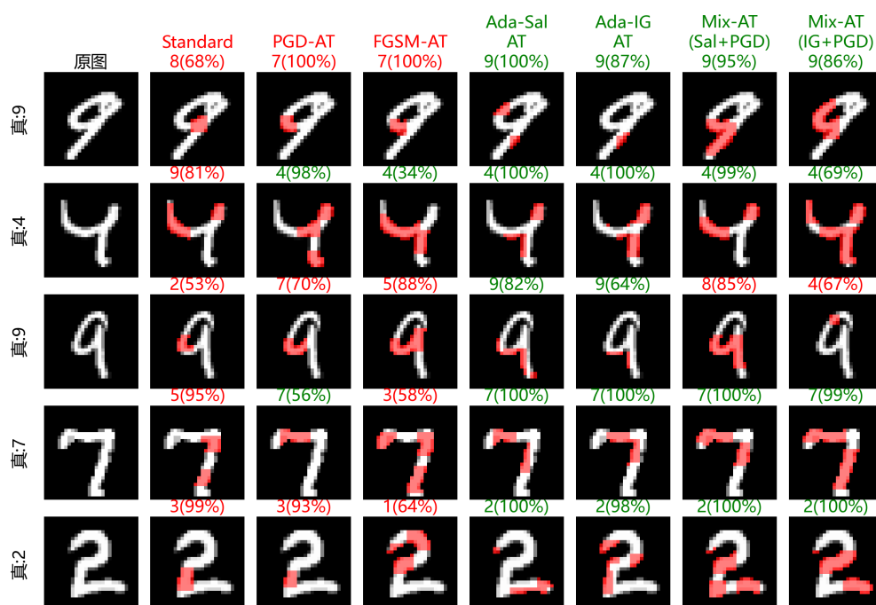
图 4.6 Adaptive-Saliency 攻击下七种模型的对比。红块为遮蔽位置；左侧为真实类别；各子图中的数字为预测类别，括号内为置信度，绿色表示预测正确，红色表示被攻破
