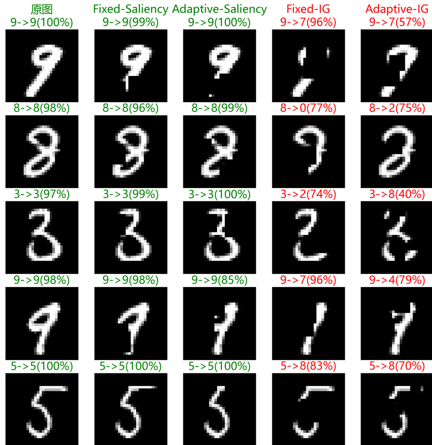
图 4.14 Adaptive-Saliency-AT 模型上四种遮蔽攻击对比。图中 a \rightarrow b(c\%) 表示真实类别、预测类别和置信度，颜色表示攻击成败
