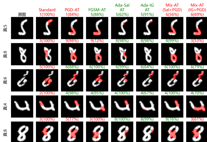
图 4.16 Fixed-Saliency 攻击下七种模型的对比。左侧为真实类别；各子图中的数字为预测类别，括号内为置信度，颜色表示预测是否正确
