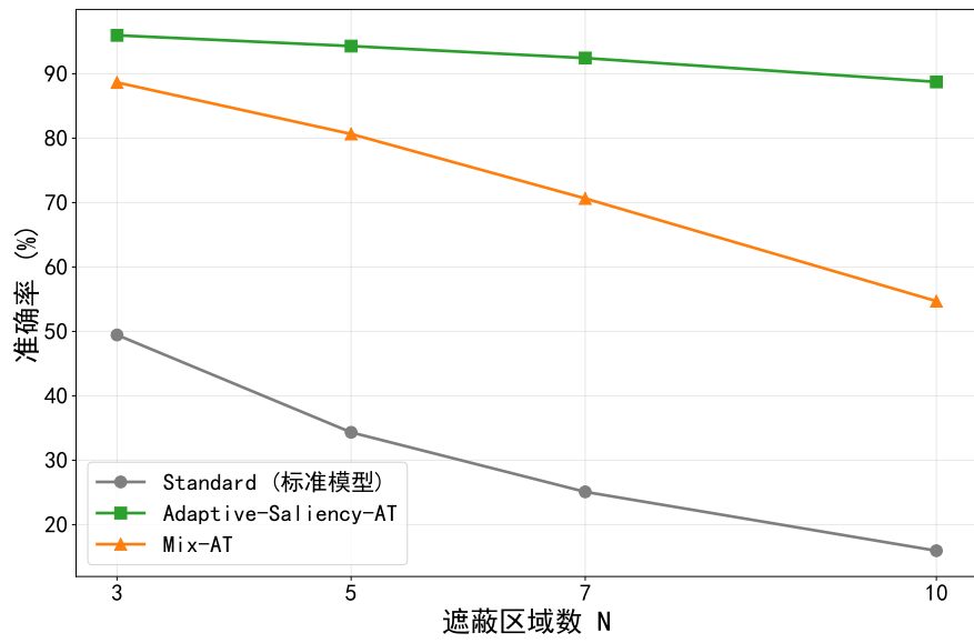
图 4.29 N 参数敏感性分析：不同防御策略下遮蔽区域数对准确率的影响 ( R = 3 )
