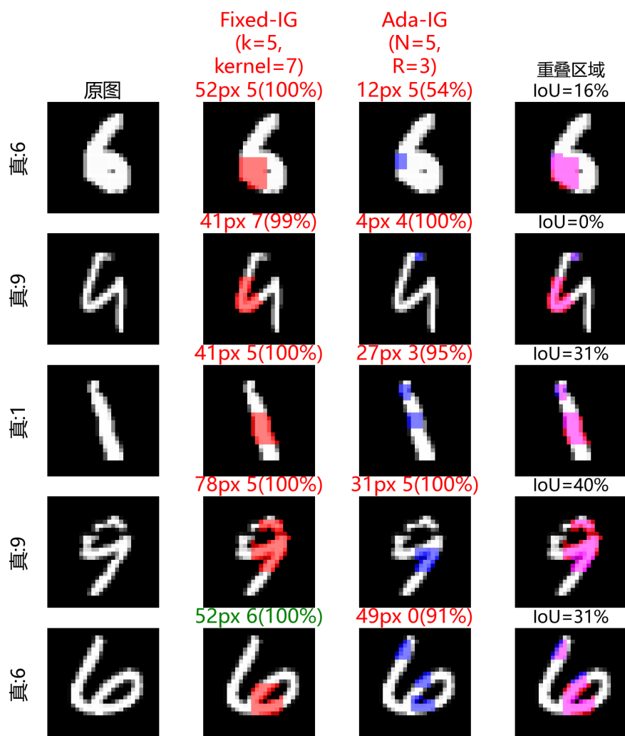
图 4.22 标准模型: Fixed-IG vs Adaptive-IG 遮挡位置对比 (参数 k = N = 5 , R = 3 , \text{kernel} = 7 )
