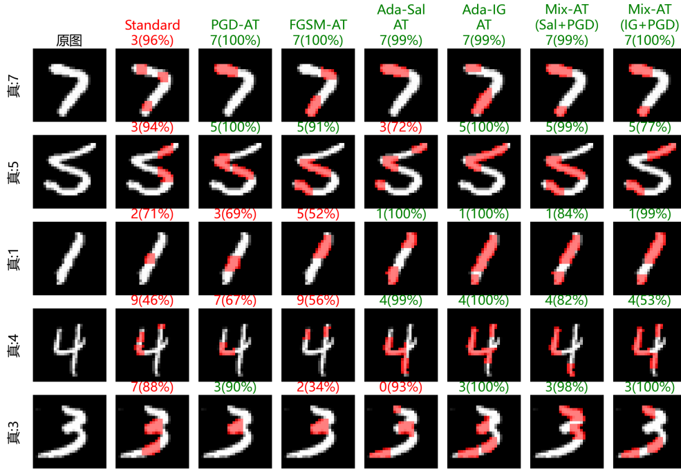
图 4.18 Adaptive-IG 攻击下七种模型的对比。左侧为真实类别；各子图中的数字为预测类别，括号内为置信度，颜色表示预测是否正确
