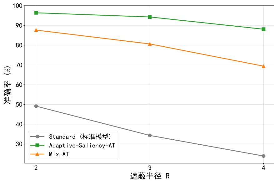
图 4.30 R 参数敏感性分析：不同防御策略下遮蔽半径对准确率的影响 ( N = 5 )
