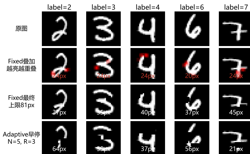
图 4.25 Fixed ( k=9, 3 \times 3 ) 与 Adaptive ( N=5, R=3 ) 遮蔽机制差异可视化。第二行红色高亮显示固定遮蔽攻击 9 个遮蔽块的累计覆盖次数，亮红色区域为多块重叠位置；第三、四行展示两种策略的最终遮蔽效果与实际像素数。固定遮蔽攻击由于显著像素空间聚集导致 52.10% 的有效面积被重叠浪费，而自适应遮蔽攻击通过逐次评估与早停以更小代价定位更分散的关键区域。
