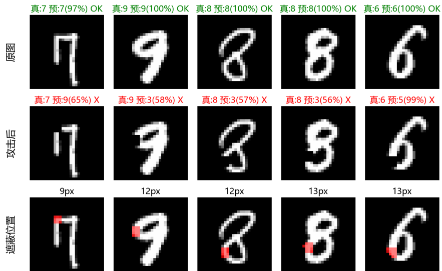
图 4.8 PGD-AT 模型上的 Adaptive-IG 攻击案例
