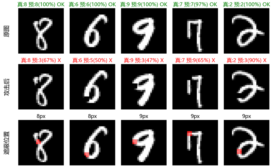
图 4.7 PGD-AT 模型上的 Adaptive-Saliency 攻击案例
