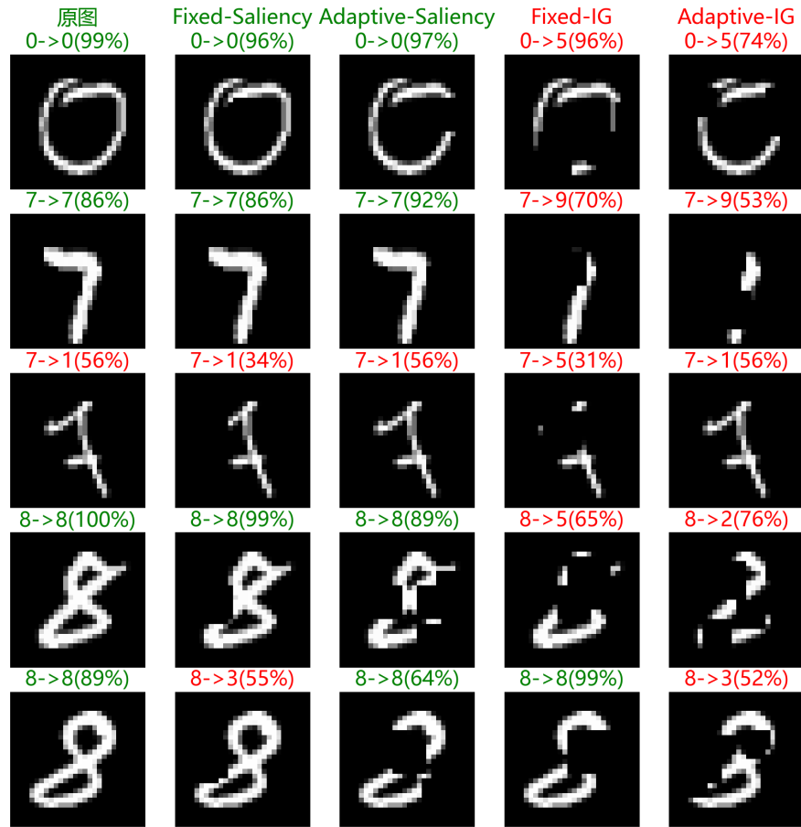
图 4.15 Adaptive-IG-AT 模型上四种遮蔽攻击对比。图中 a \rightarrow b(c\%) 表示真实类别、预测类别和置信度，颜色表示攻击成败
