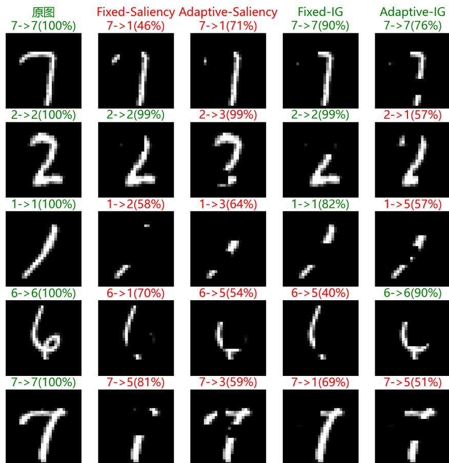
图 4.13 PGD-AT 模型上四种遮蔽攻击对比。图中 a \rightarrow b(c\%) 表示真实类别、预测类别和置信度，颜色表示攻击成败
