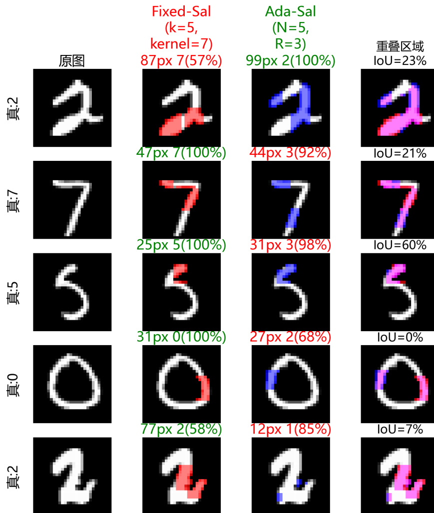
图 4.21 标准模型: Fixed-Saliency vs Adaptive-Saliency 遮蔽位置对比
