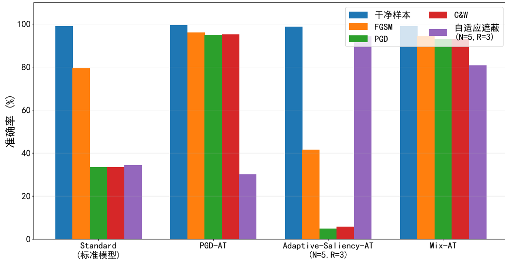
图 4.26 各防御策略在不同攻击类型下的准确率对比
