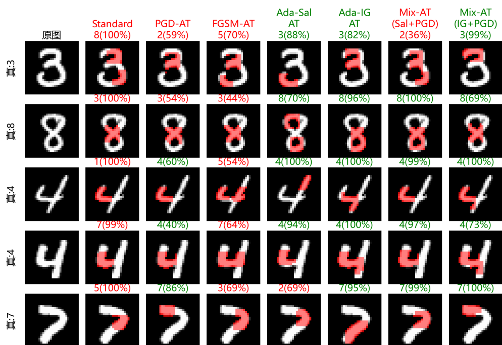
图 4.17 Fixed-IG 攻击下七种模型的对比。左侧为真实类别；各子图中的数字为预测类别，括号内为置信度，颜色表示预测是否正确
