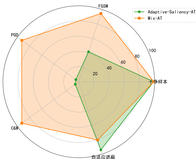
图 4.27 Adaptive-Saliency-AT 与 Mix AT 综合性能雷达图对比
