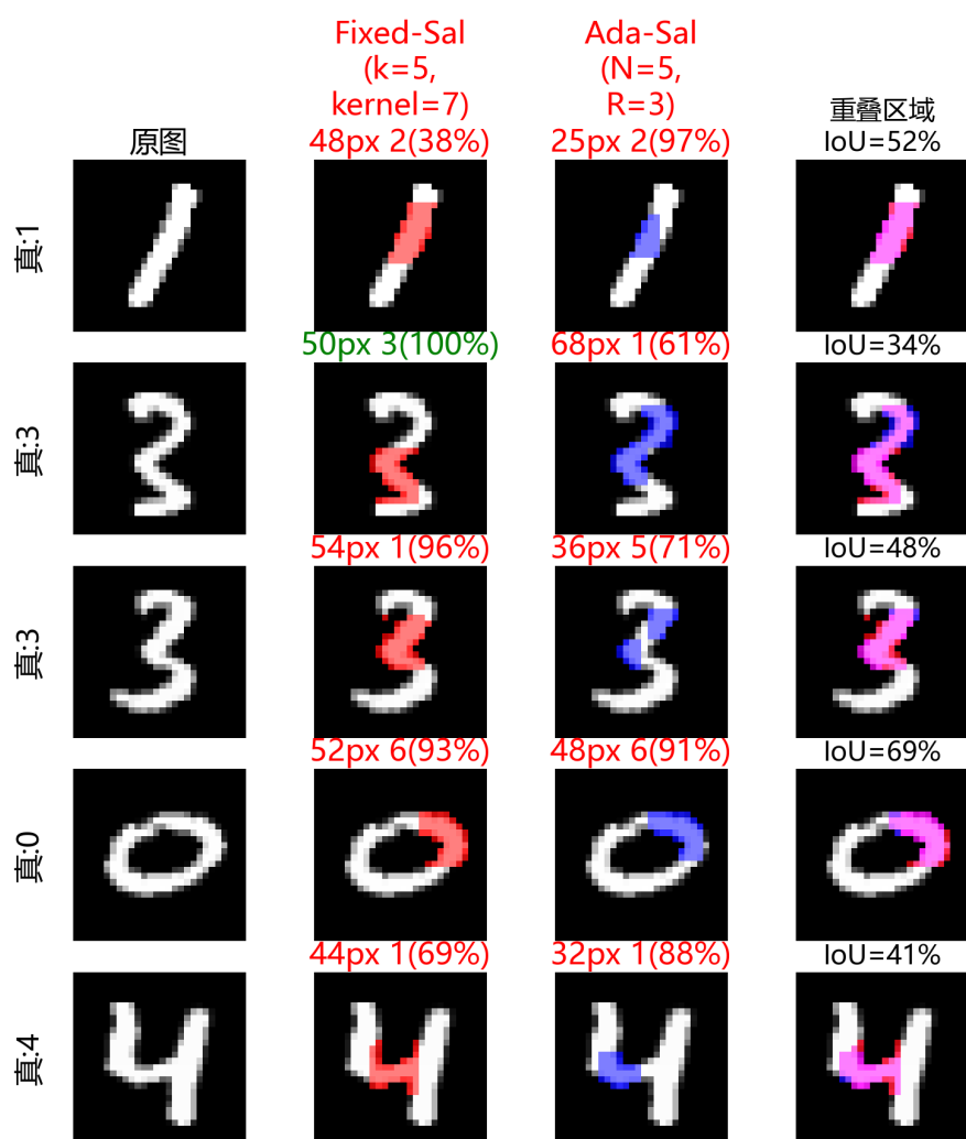
图 4.23 PGD-AT 模型: Fixed-Saliency vs Adaptive-Saliency 遮蔽位置对比
