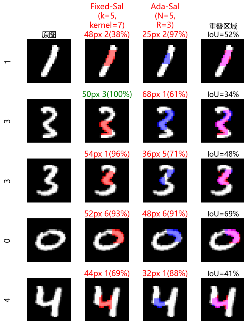
图 4.23 PGD-AT 模型: Fixed-Saliency vs Adaptive-Saliency 遮蔽位置对比
