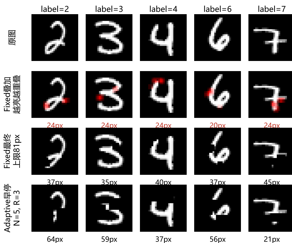
图 4.25 Fixed ( k=9, 3 \times 3 ) 与 Adaptive ( N=5, R=3 ) 遮蔽机制差异可视化。第二行红色高亮显示固定遮蔽攻击 9 个遮蔽块的累计覆盖次数，亮红色区域为多块重叠位置；第三、四行展示两种策略的最终遮蔽效果与实际像素数。固定遮蔽攻击由于显著像素空间聚集导致 52.10% 的有效面积被重叠浪费，而自适应遮蔽攻击通过逐次评估与早停以更小代价定位更分散的关键区域。
