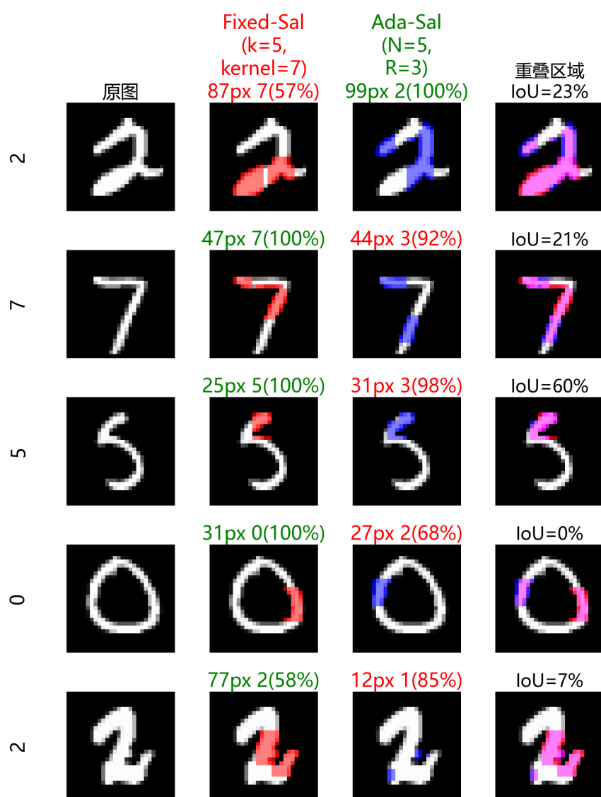
图 4.21 标准模型：Fixed-Saliency vs Adaptive-Saliency 遮蔽位置对比
