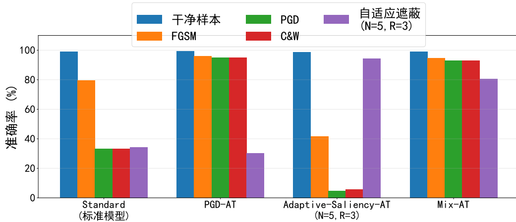
图 4.26 各防御策略在不同攻击类型下的准确率对比
