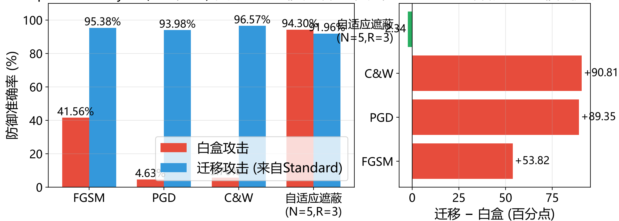
Adaptive-Saliency-AT(N=5,R=3) 在白盒 vs 迁移攻击下的准确率 差距: >0 意味着白盒比迁移更脆弱
