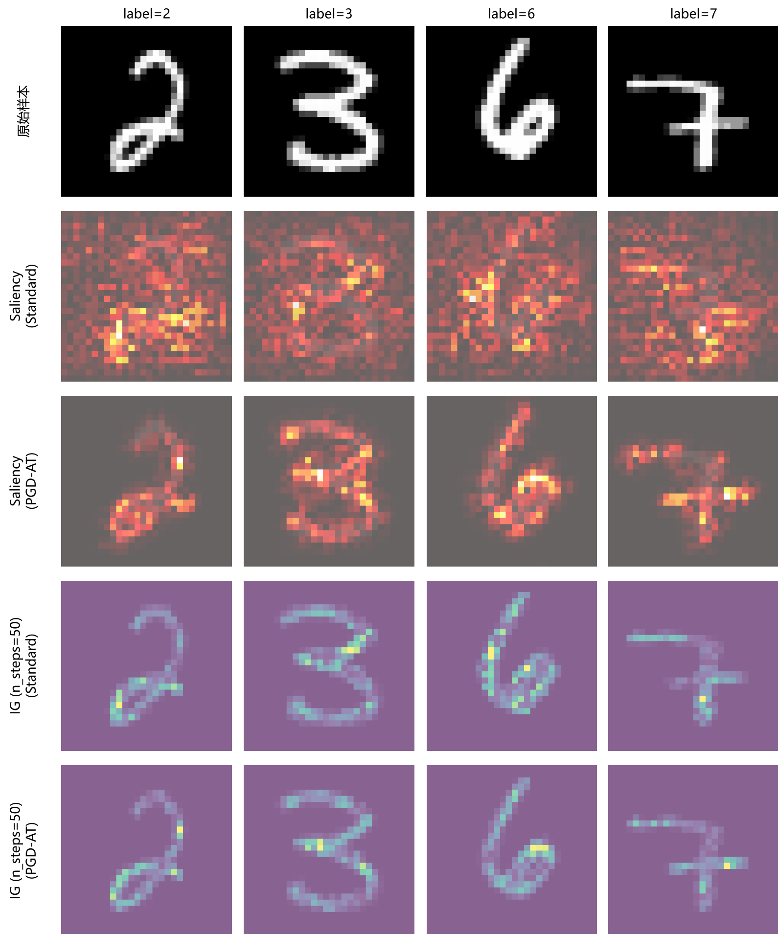
两种归因方法在 Standard 与 PGD-AT 模型上的差异——PGD-AT 使 IG 归因更分散（梯度掩蔽对路径积分的系统性干扰）
