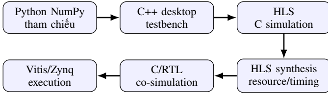
Fig. 4. Luồng kiểm chứng nhiều tầng được sử dụng trong dự án.
