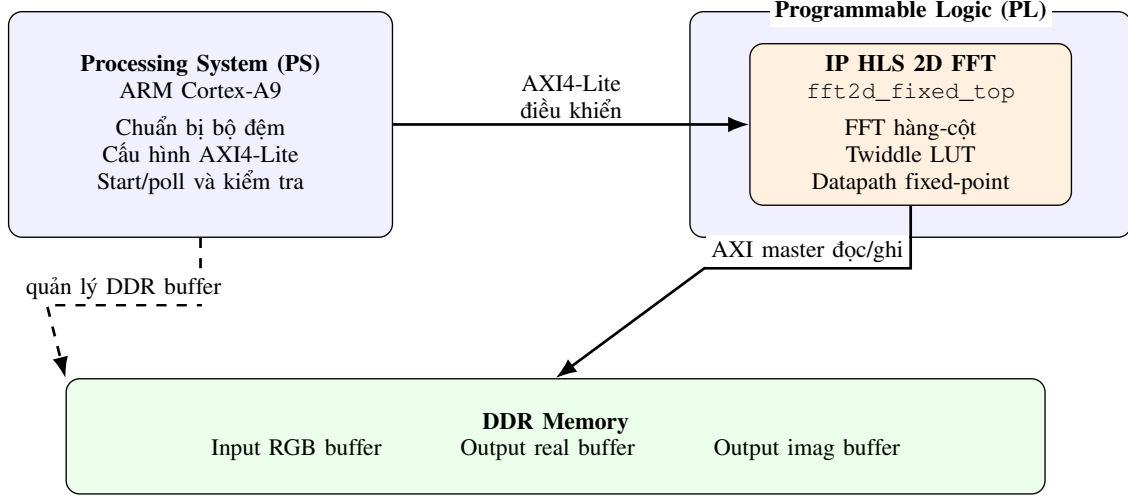
Fig. 1. Kiến trúc tổng quan của bộ tăng tốc 2D FFT trên Zynq.
