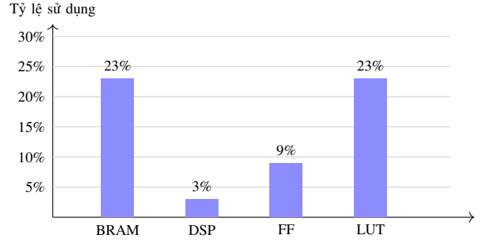
Fig. 5. Biểu đồ tỷ lệ sử dụng tài nguyên của thiết kế trên xc7z020clg400-1.
