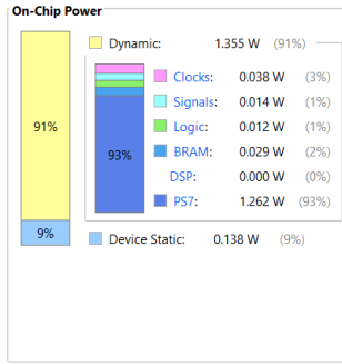
Hình 14. Báo cáo công suất sau triển khai.
