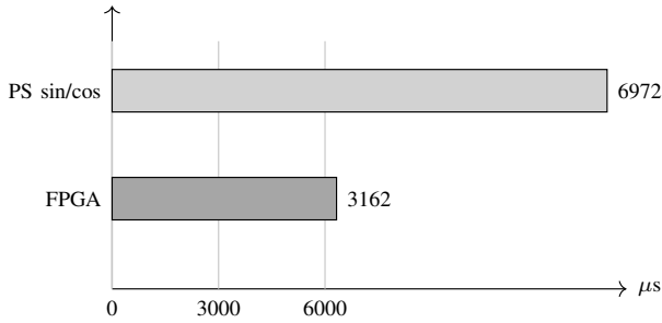
Hình 17. Thời gian trung bình trên board.
