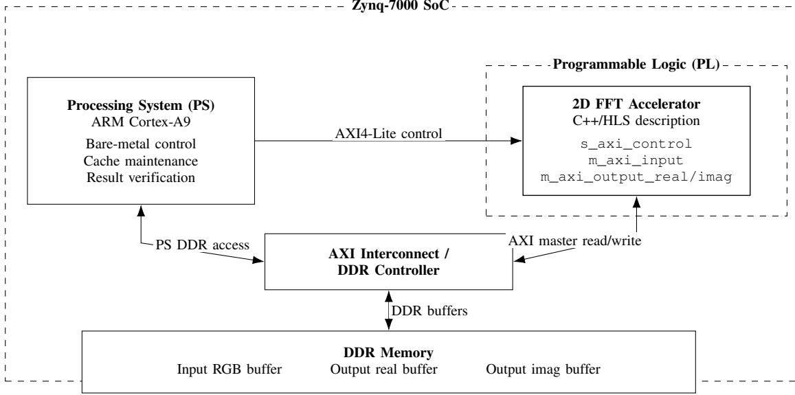
Hình 2. Kiến trúc hệ thống.
