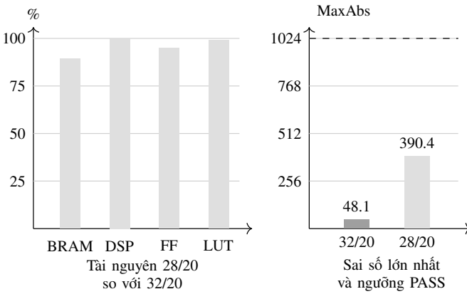
Hình 10. Đánh đổi độ rộng bit fixed-point.
