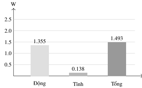
Hình 15. So sánh công suất on-chip.
