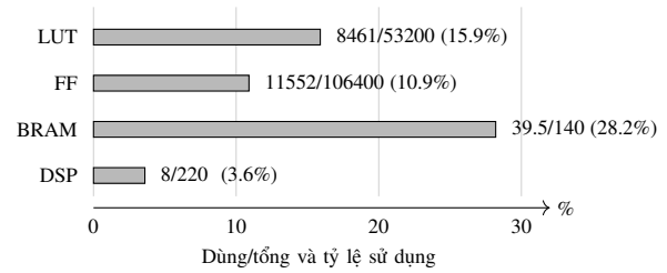
Hình 12. Biểu đồ chi tiết tài nguyên sau triển khai.
