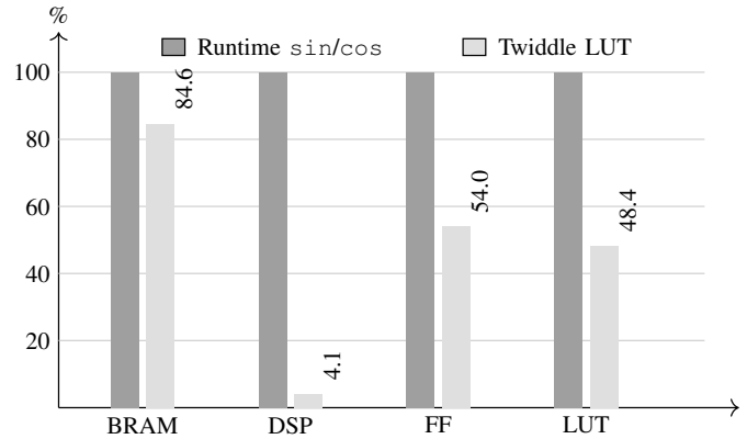
Hình 7. Tỷ lệ tài nguyên sau tối ưu bằng bảng tra twiddle.
