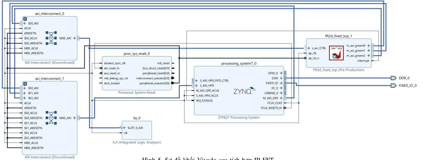
Hình 5. Sơ đồ khối Vivado sau tích hợp IP FFT.
