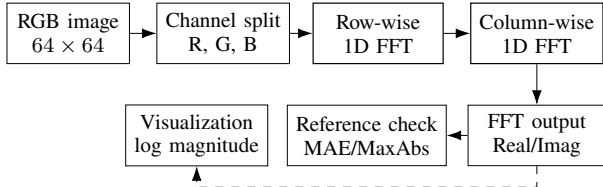
Hình 3. Luồng xử lý ảnh RGB.
