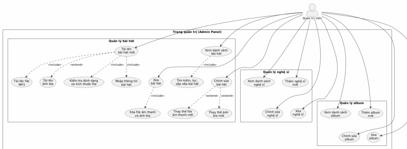
Sơ đồ Use Case: Quản trị hệ thống
