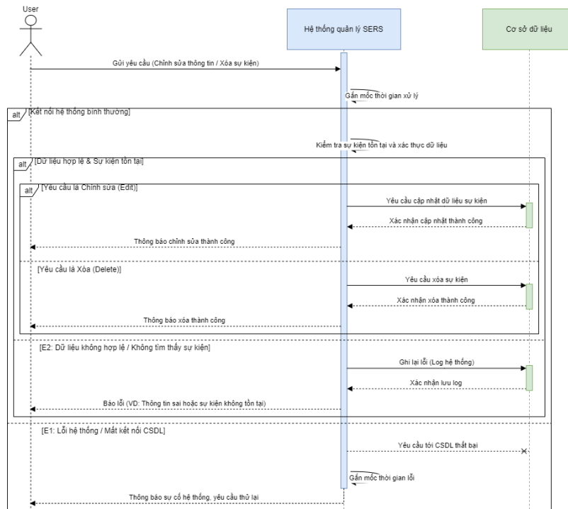
Hình 2: Sequence Diagram (EDit/Delete Event) mô tả cho việc chỉnh sửa và xóa event
