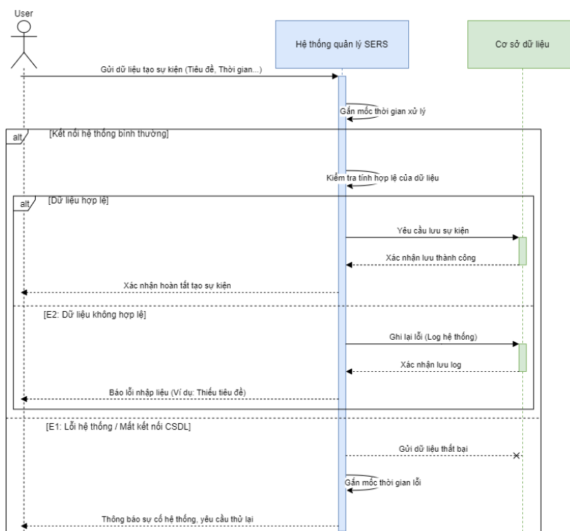
Hình 1: Sequence Diagram (Create Event) mô tả cho việc tạo mới event
