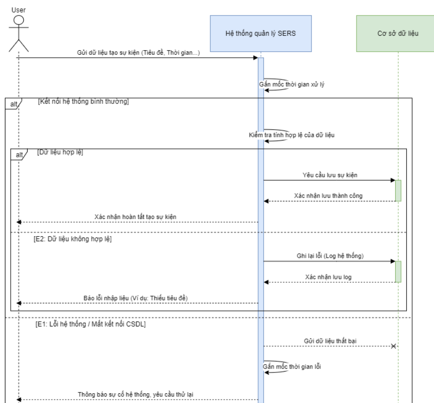
Hình 1: Sequence Diagram mô tả cho việc tạo mới event
