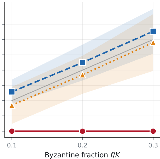
Gradient scaling
