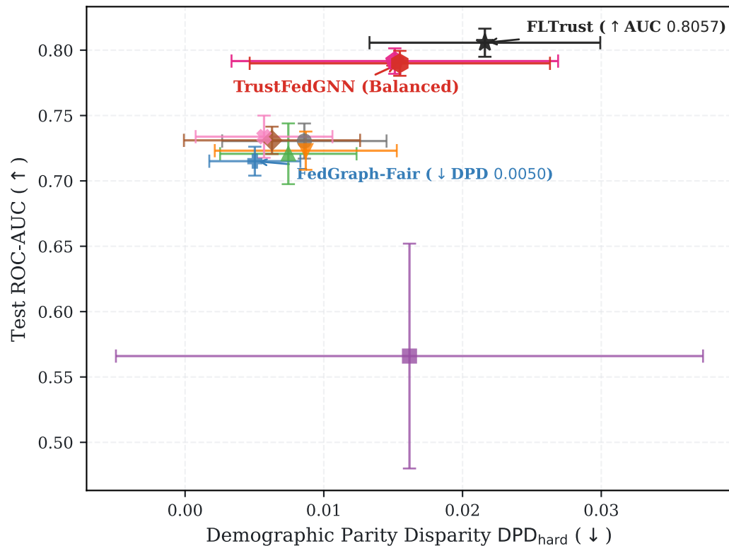
Pareto Frontier: Pokec-z ( N = 67,796 )
