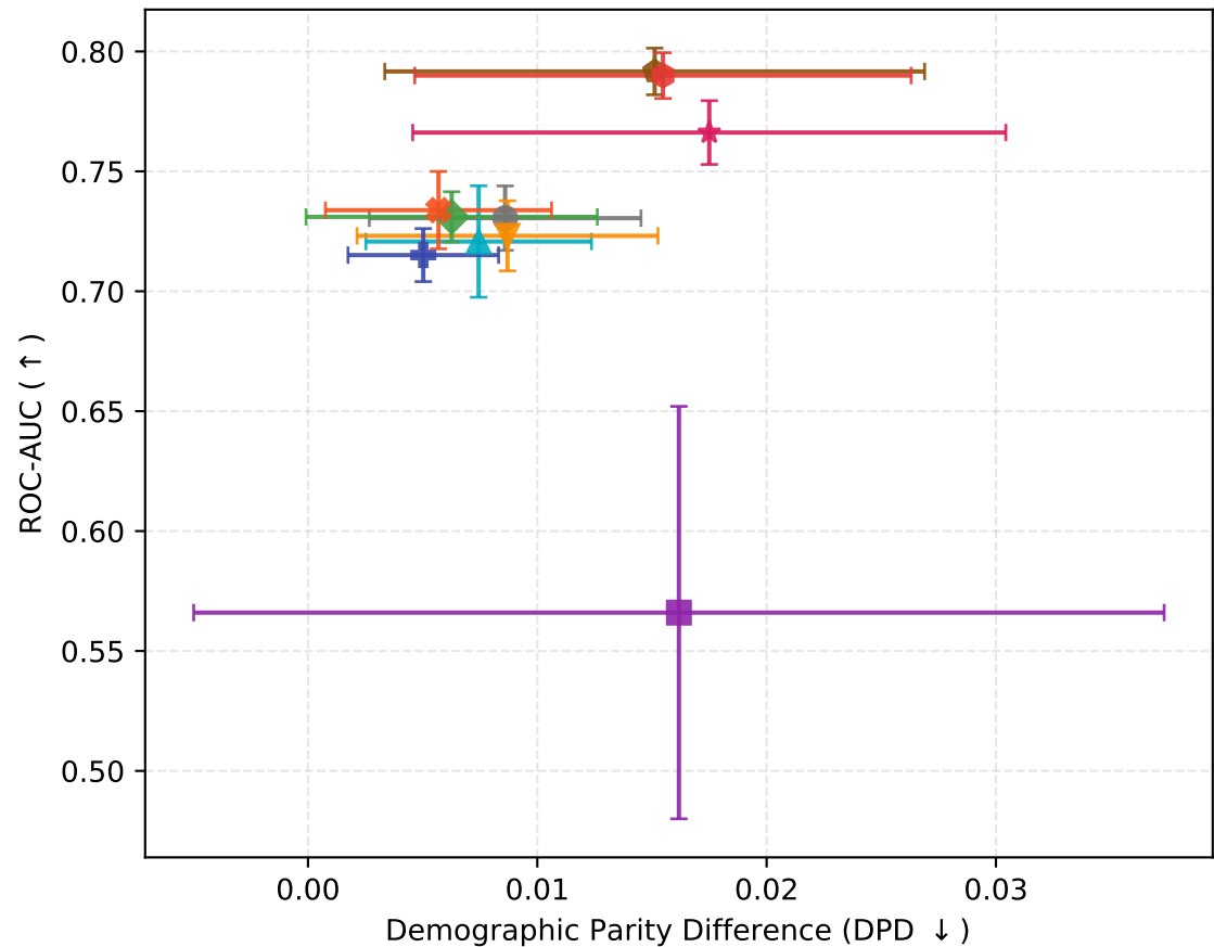
Pareto Frontier: Pokec-z
