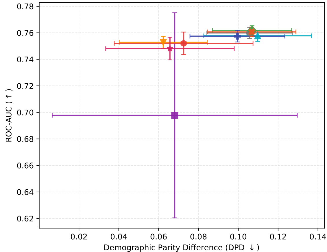
Pareto Frontier: Credit Default
