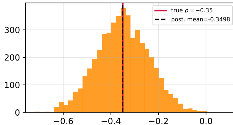
MALA posterior: \rho
