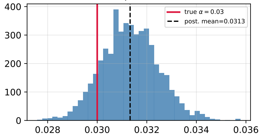
MALA posterior: \alpha
