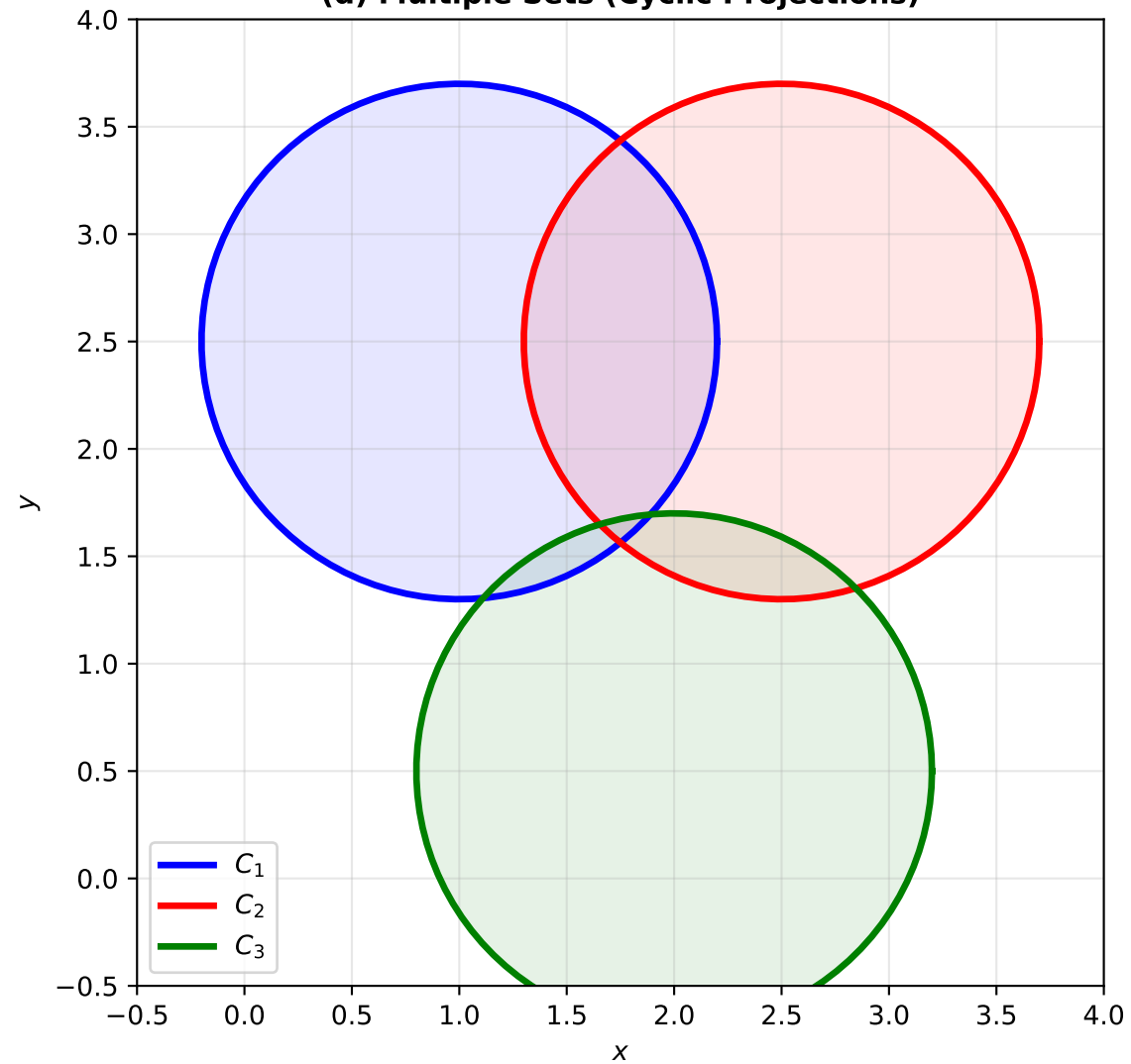
(d) Multiple Sets (Cyclic Projections)
