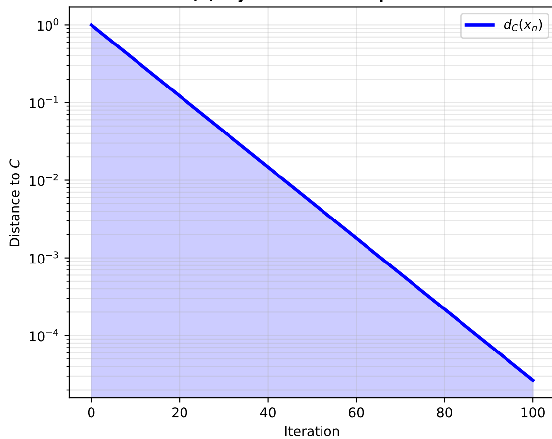
(d) Fejér Monotone Sequence
