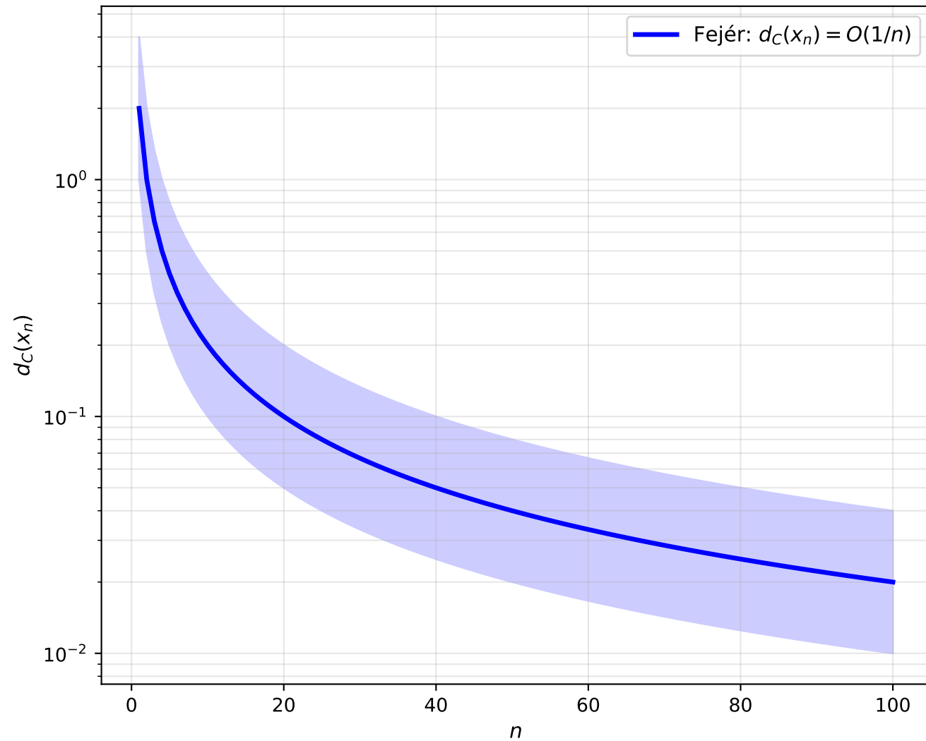
(a) Exact Fejér Monotonicity
