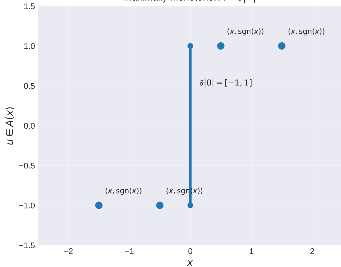
Maximally Monotone: A = \partial|\cdot|
