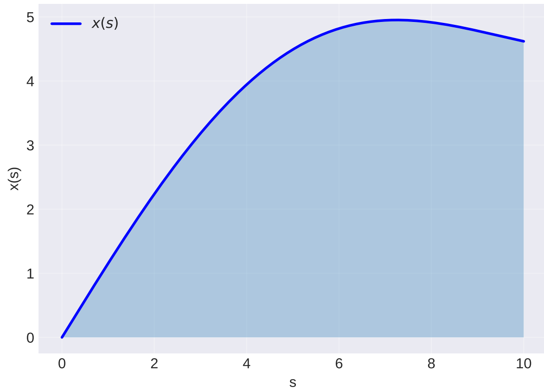
Input Function x(s)
