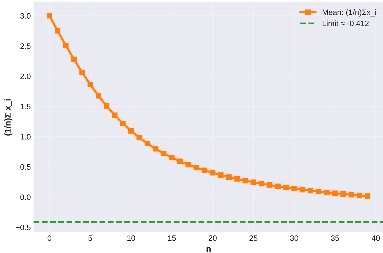
Mean Convergence (Cesàro Averaging)
