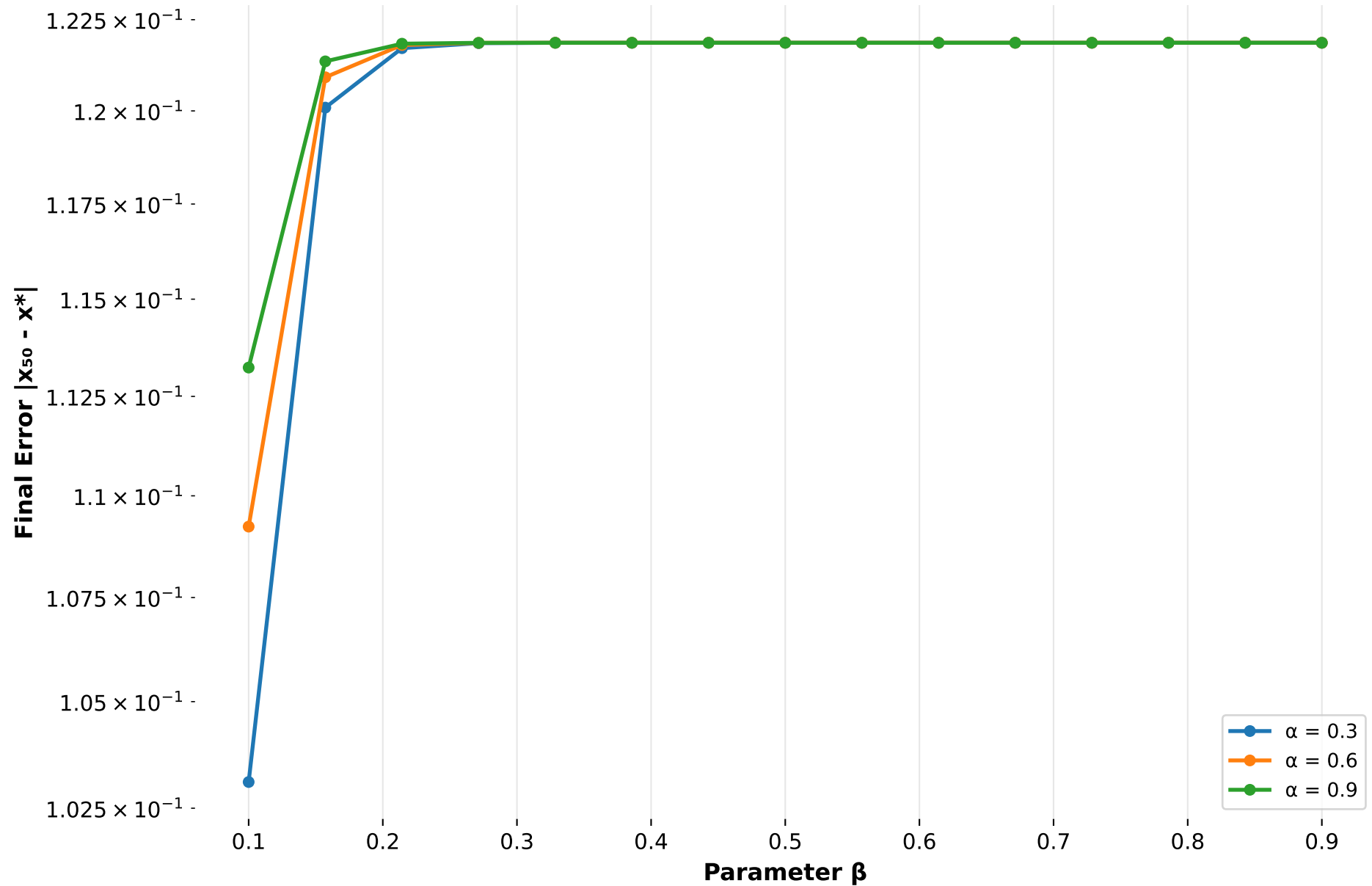
Parameter Effect on Ishikawa Iteration
