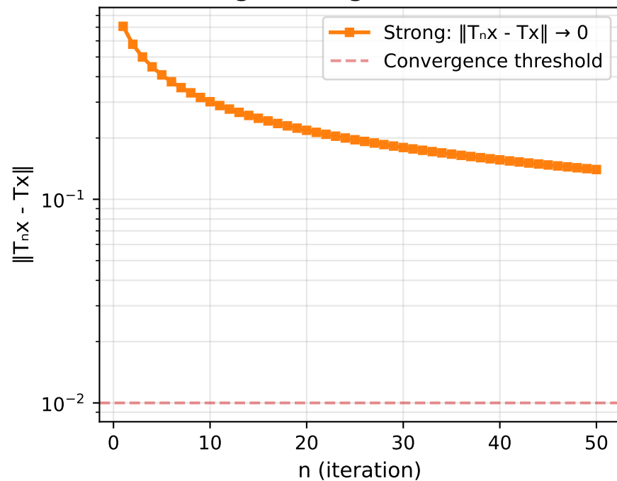
Strong Convergence (Medium)
