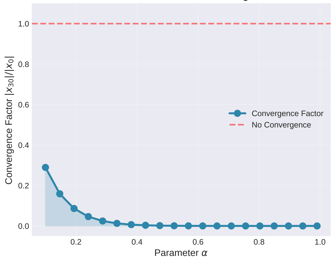
Parameter Influence on Convergence
