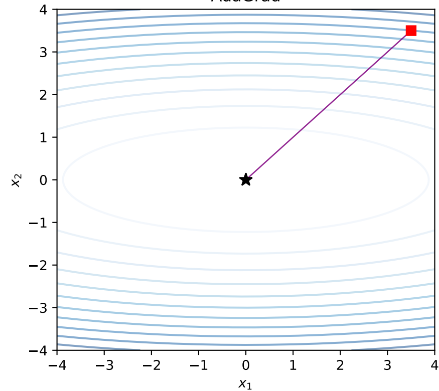
AdaGrad
