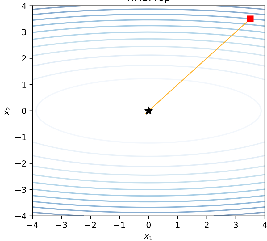
RMSProp
