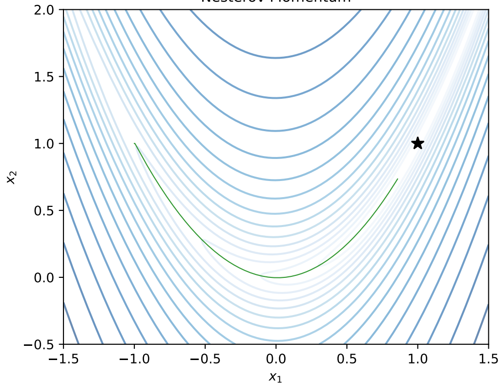
Nesterov Momentum
