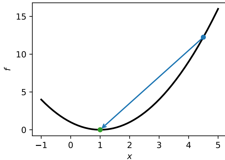
Convergence (quadratic)
