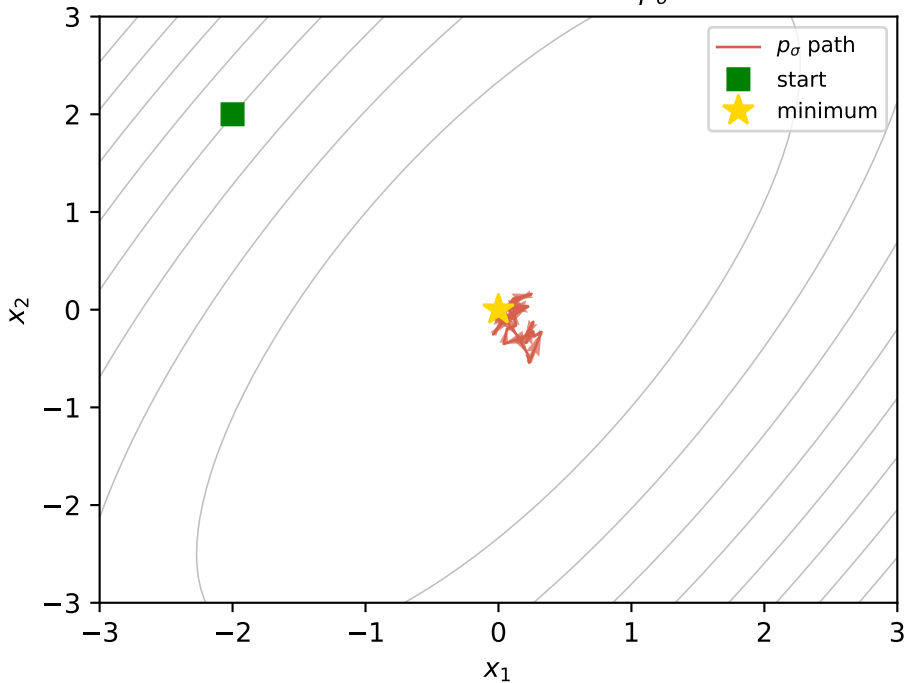
CMA-ES Evolution Path p_\sigma
