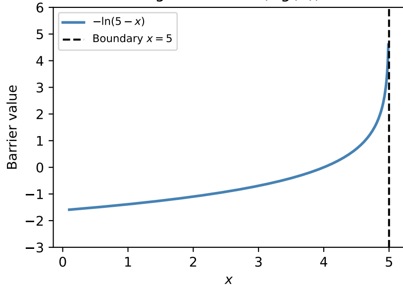
Log Barrier: -\ln(-g(\mathbf{x}))
