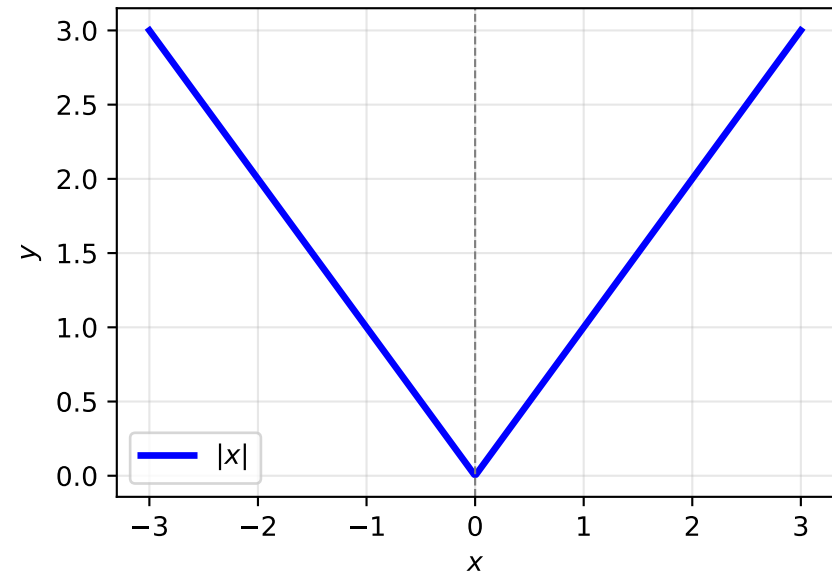
Absolute Value |x|
