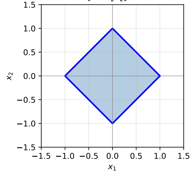
L_1 ball \|\mathbf{x}\|_1 \leq 1
