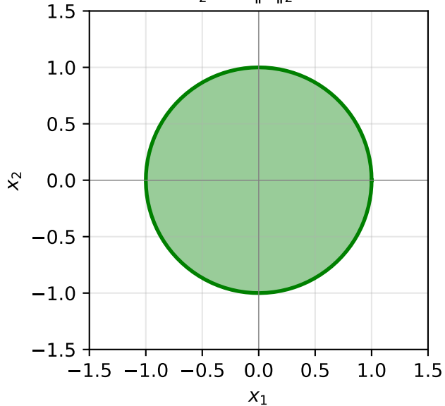
L_2 ball \|\mathbf{x}\|_2 \leq 1
