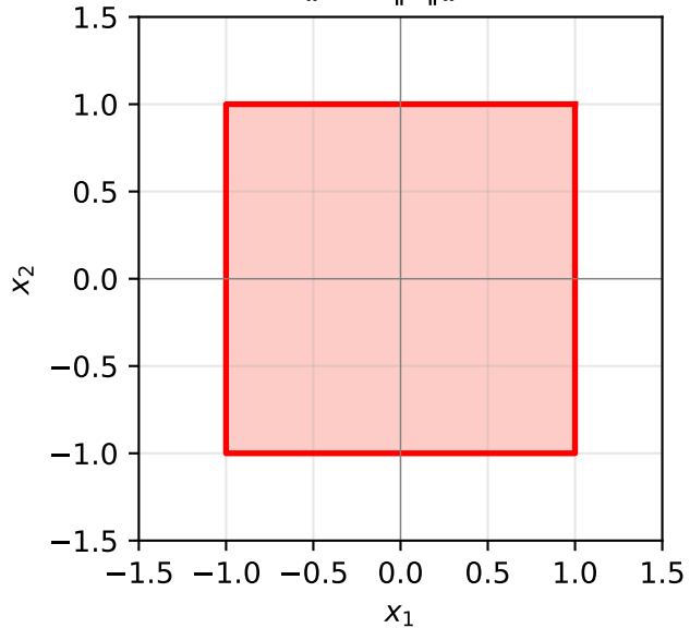
L_\infty ball \|\mathbf{x}\|_\infty \leq 1
