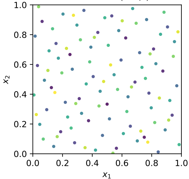
Halton n=100 (b=2,3)
