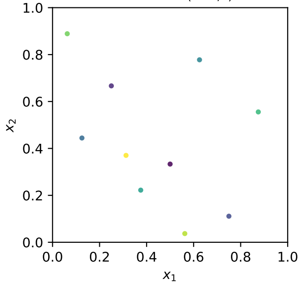
Halton n=10 (b=2,3)
