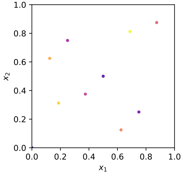
Sobol n=10
