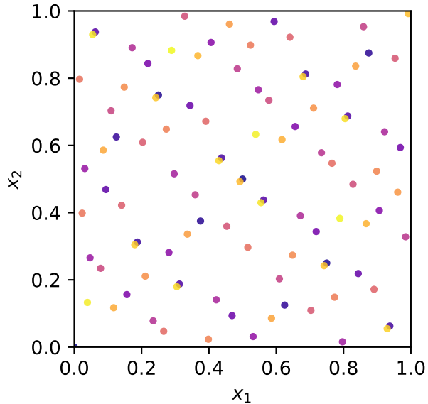
Sobol n=100
