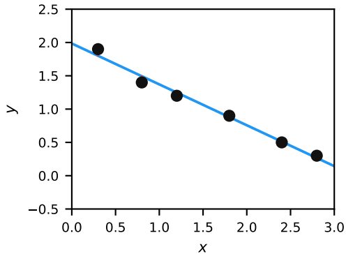
m > n + 1
