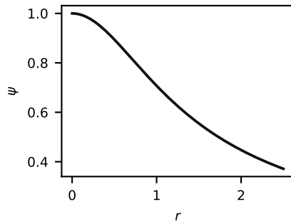
inv. multiquadratic: (r^2 + \sigma^2)^{-1/2}
