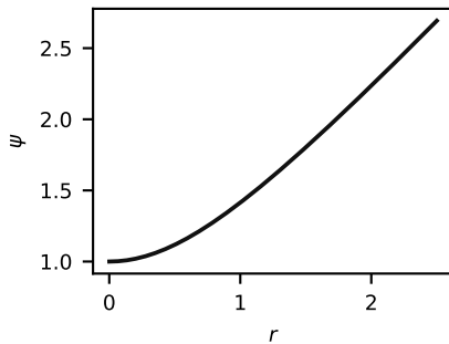
multiquadratic: (r^2 + \sigma^2)^{1/2}
