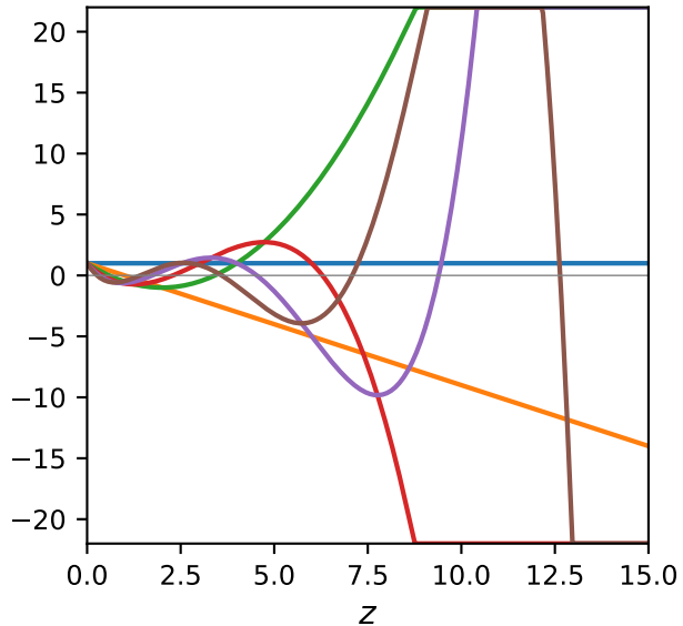
Laguerre
