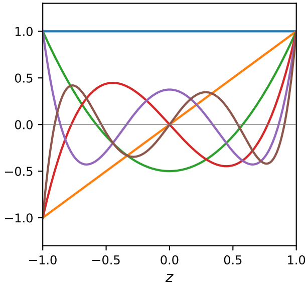
Legendre
