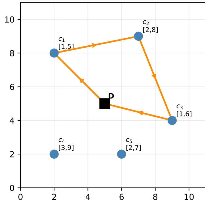
Step 2: Insert c_1 to get D- c_1 - c_2 - c_3 -D
