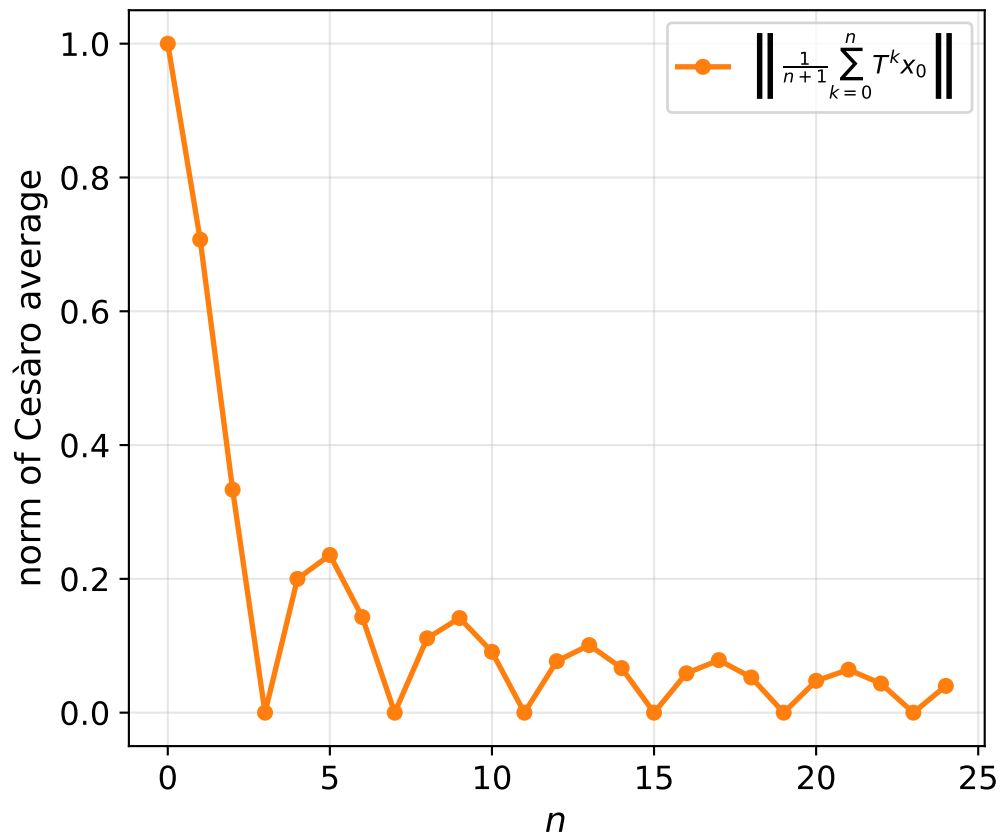
Baillon: Cesàro averages converge to Fix T
