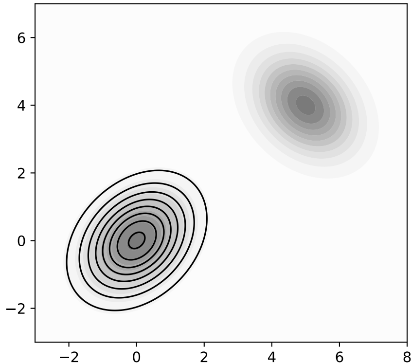
Minimize KL(Q\|P)
