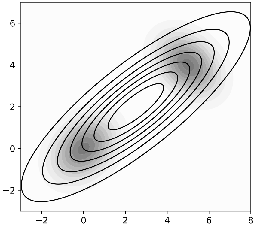
Minimize KL(P\|Q)
