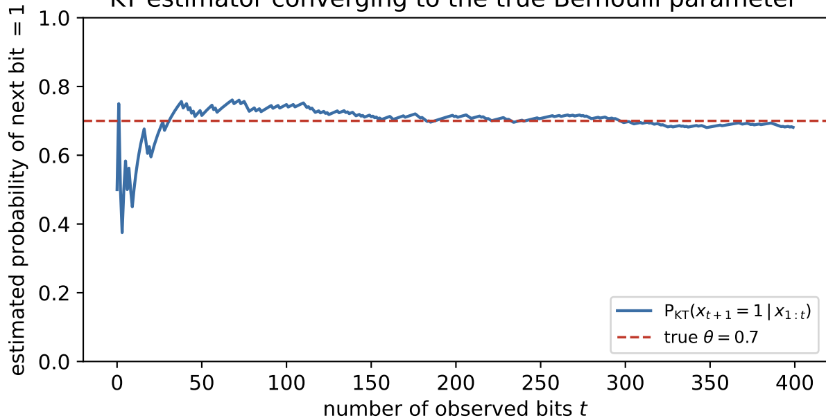
KT estimator converging to the true Bernoulli parameter
