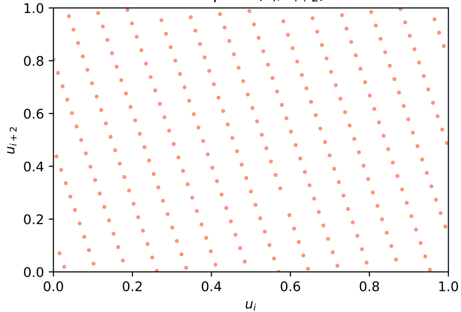
LCG pairs (u_i, u_{i+2})
